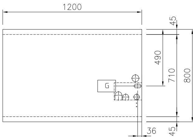
Boven aanzicht
